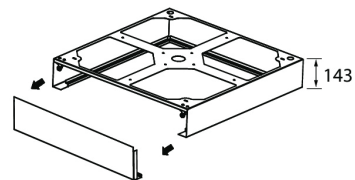
Pinta-asennuskehys.
