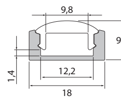
Slimline 7 optinen 60°
